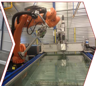
cellule de CND de pièces composites A350 (Stélia, Airbus Group)
