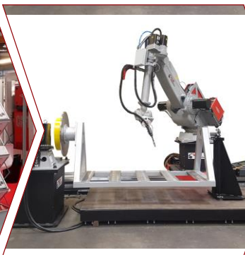
cellule de fabrication additive métal pièces > 5 m (Polyshape)
